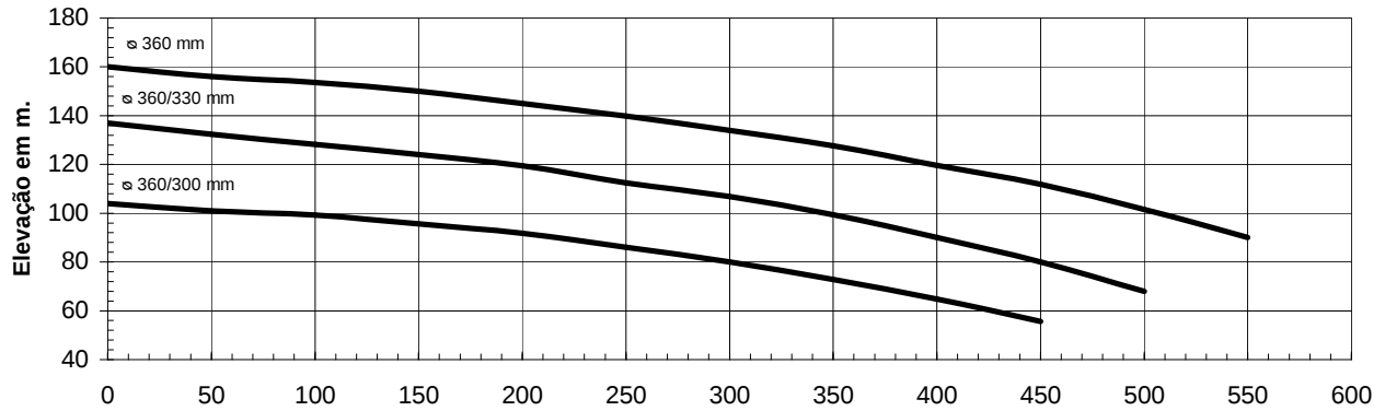
Curva para 2 estágios
